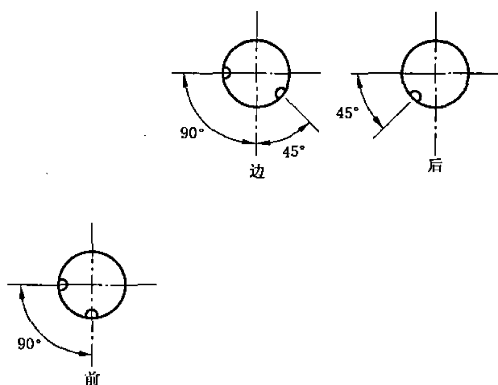
图 B.2 方形点火器各边的截面图
