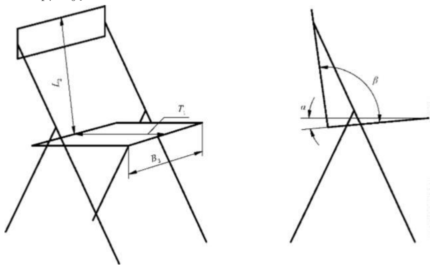
图 4 折叠椅尺寸示意图
