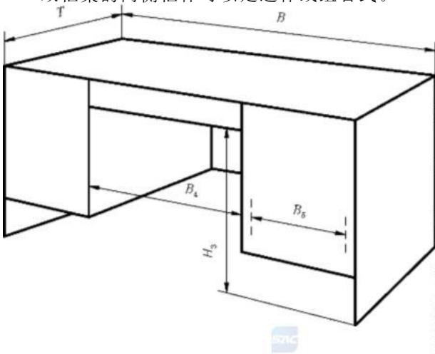
图 8 双柜桌尺寸示意图
