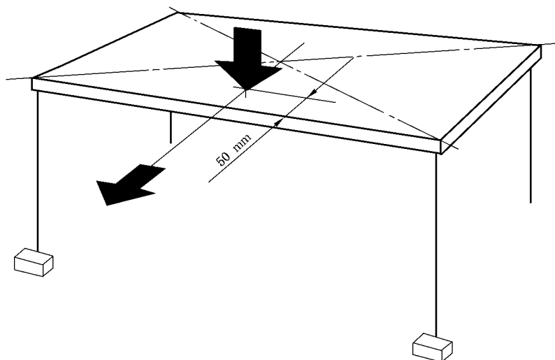
图 1 桌类稳定性加载试验
