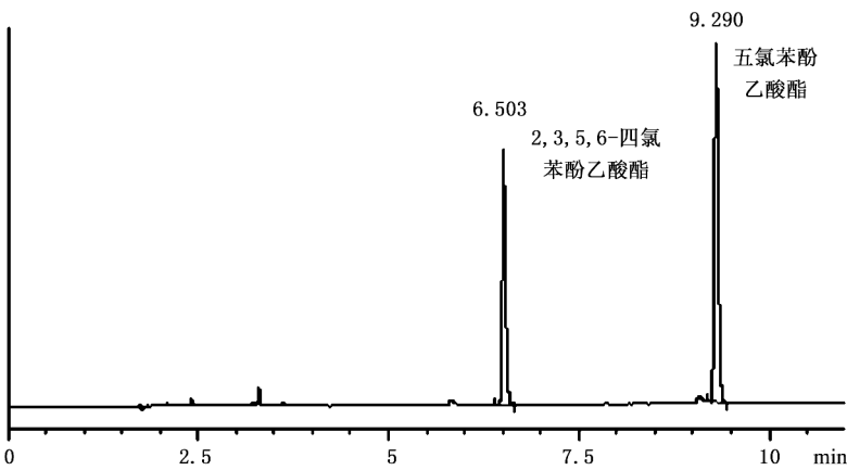
图 B.1 五氯苯酚(PCP)乙酸酯和 2,3,5,6-四氯苯酚(TeCP)乙酸酯标准物气相色谱图
