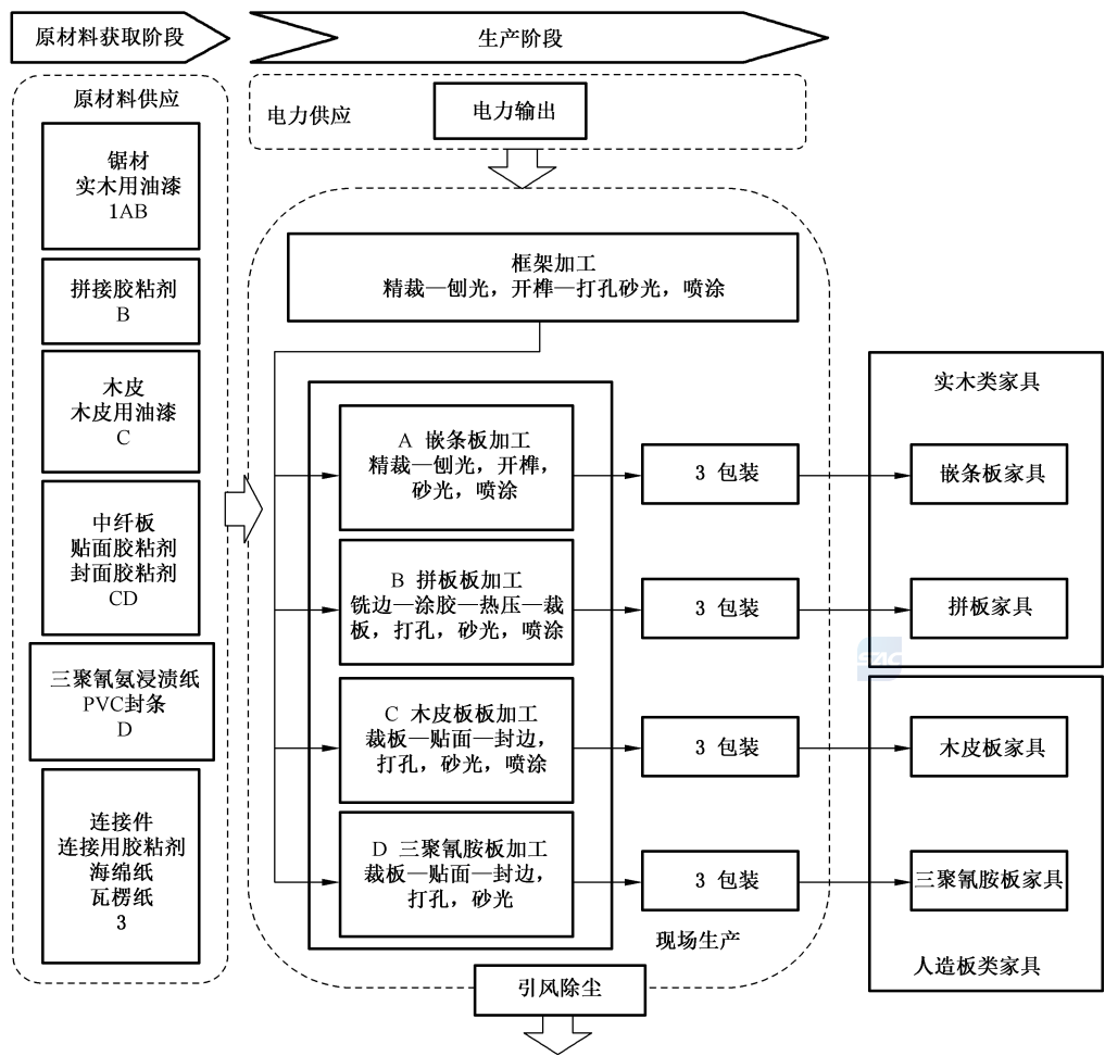
图 B.1 木制家具产品系统边界
