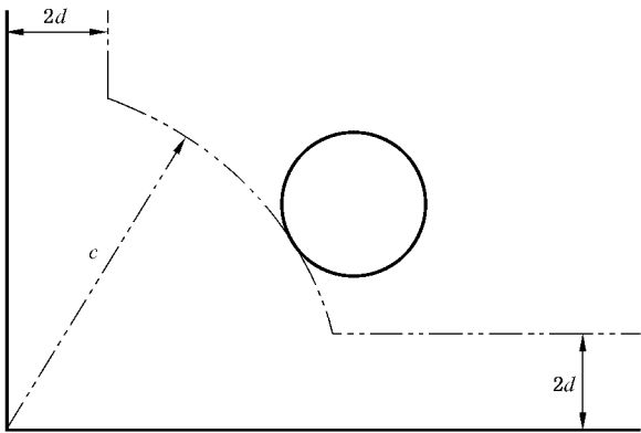
图 3 孔的边部距玻璃角部的距离示意图
