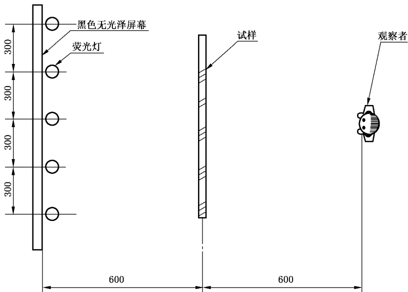
图 2 针孔、斑点、划伤的测定示意图
