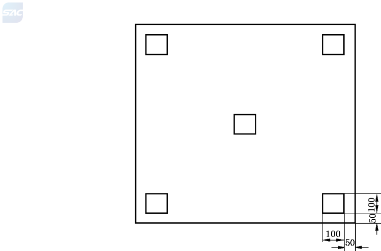
图 4 取样位置
