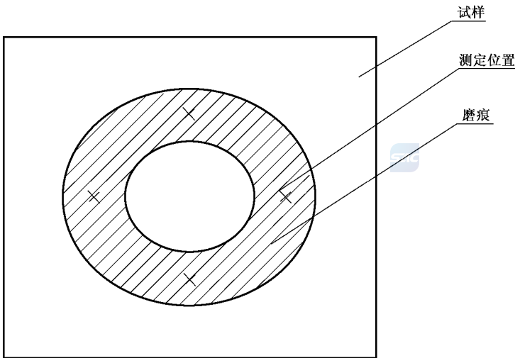
图 5 测定位置
