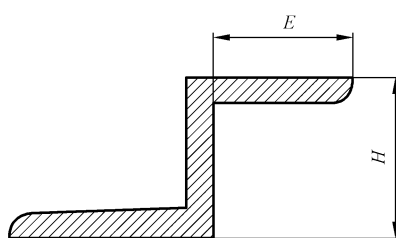
图 14 横截面尺寸图示 12
