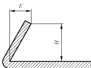
图 13 横截面尺寸图示 11
