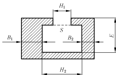
图 6 横截面尺寸图示 4
