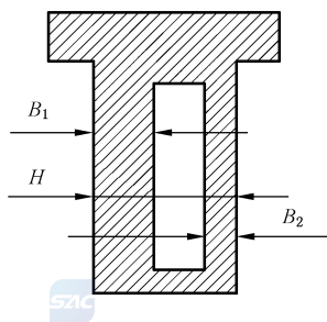
图 3 横截面尺寸图示 1
