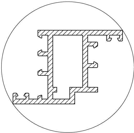
图 1 外接圆示意图
