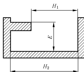
图 6 横截面尺寸图示 4
