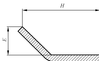
图 12 横截面尺寸图示 10
