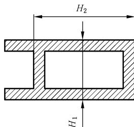
图 5 横截面尺寸图示 3
