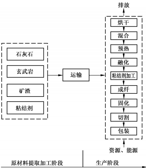
图 C.2 岩棉板的工艺流程图
