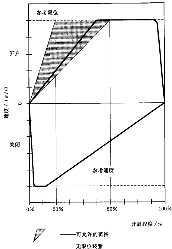
图 2 非平开门/窗的试验周期
