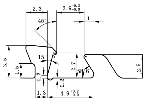
图 C.1 穿条型材槽口示意图
