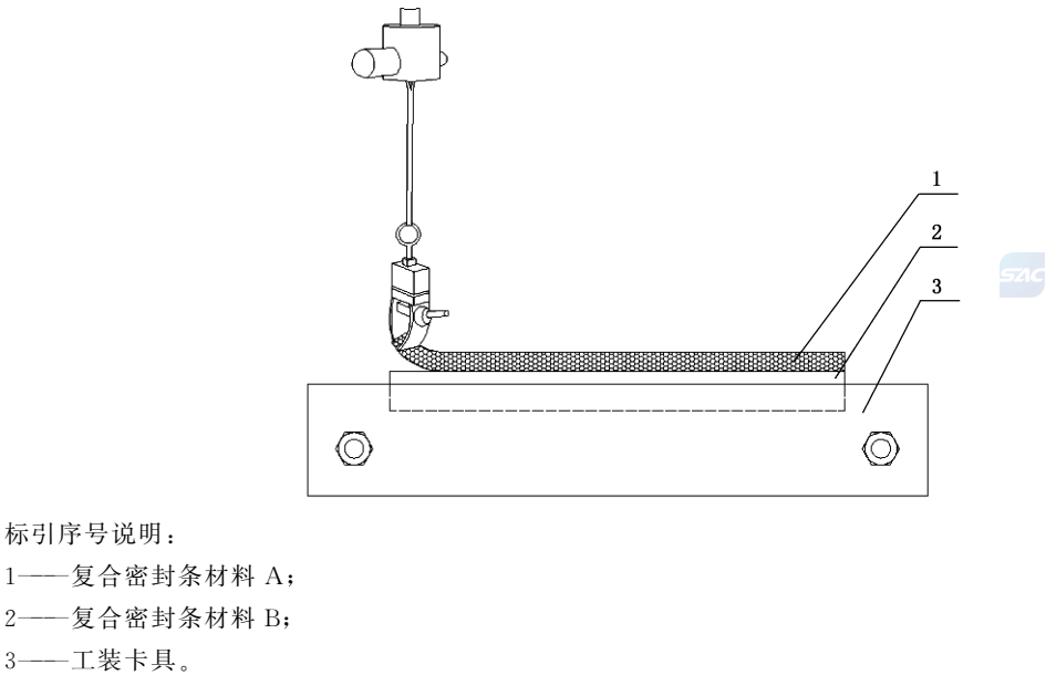
图 2 抗剥离性试验示意图
